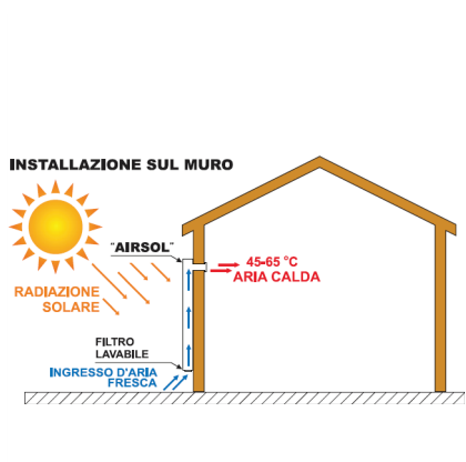
INSTALLAZIONE SUL MURO:
