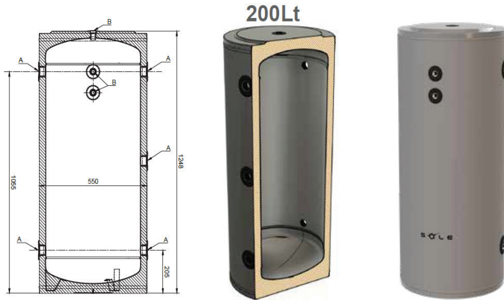
BF 200 / SEZIONE TRASVERSALE
