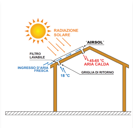
INSTALLAZIONE SUL TETTO:
